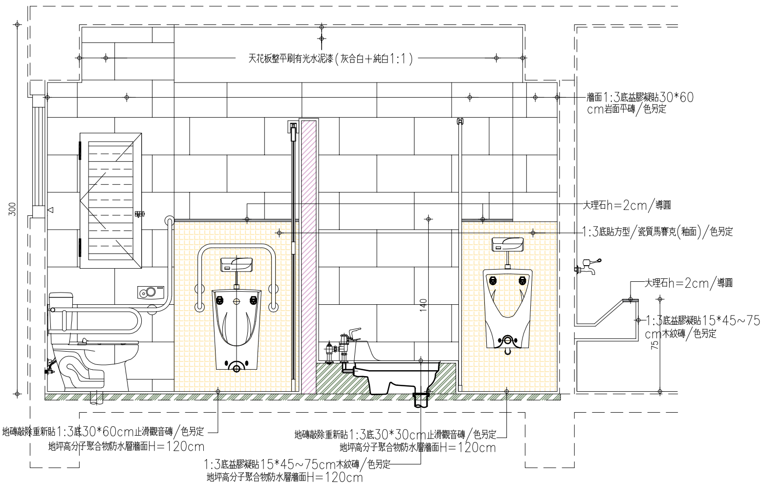
2 F—F剖面圖 A1:S=1/15 A3:S=1/30
